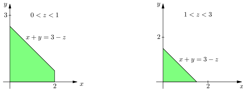
Figura 4: Cortes em W perpendiculares a Oz
