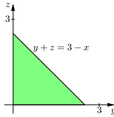
Figura 5: Corte em W perpendicular a Ox
