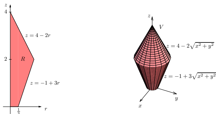
Figura 1: O conjunto V obtém-se rodando a região plana R em torno do eixo Oz
