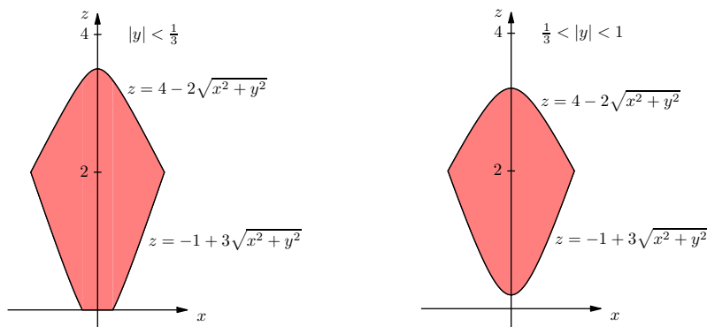
Figura 2: Cortes em V perpendiculares a Oy
