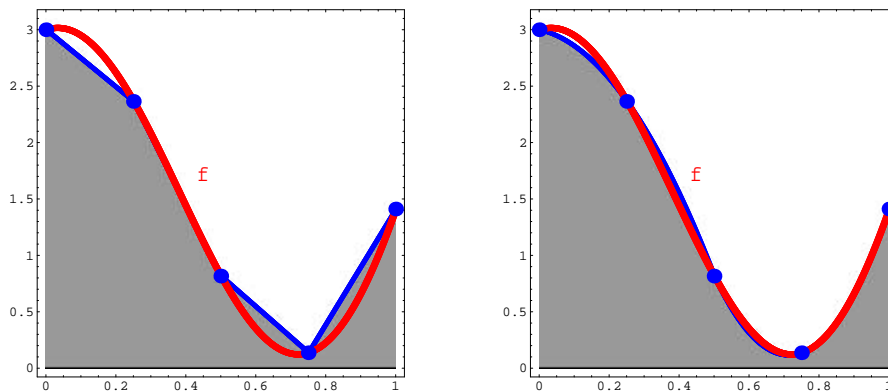
Figura 1: Aplicação das regras dos trapézios composta e de Simpson composta.
